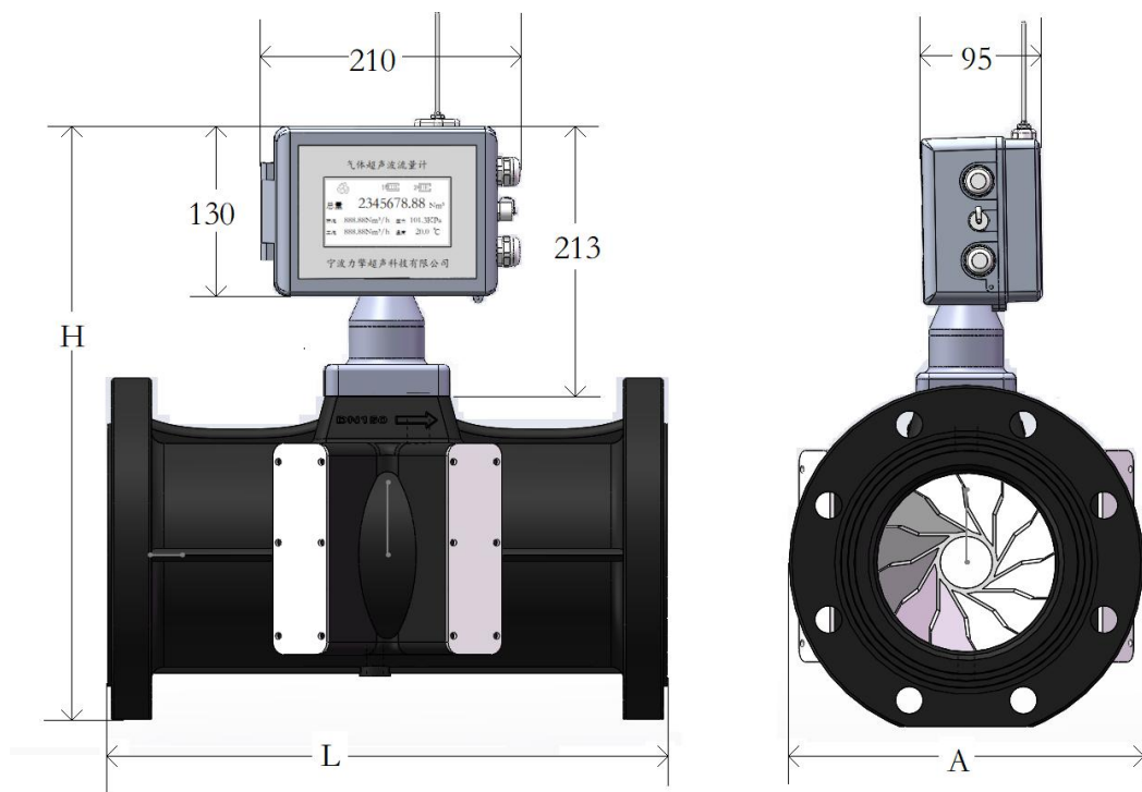
图5 LQUA 气体超声流量计（四声道）外形尺寸图
