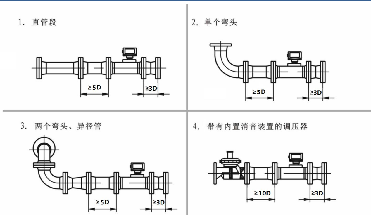
图 9 LQUA 气体超声流量计推荐安装方式
