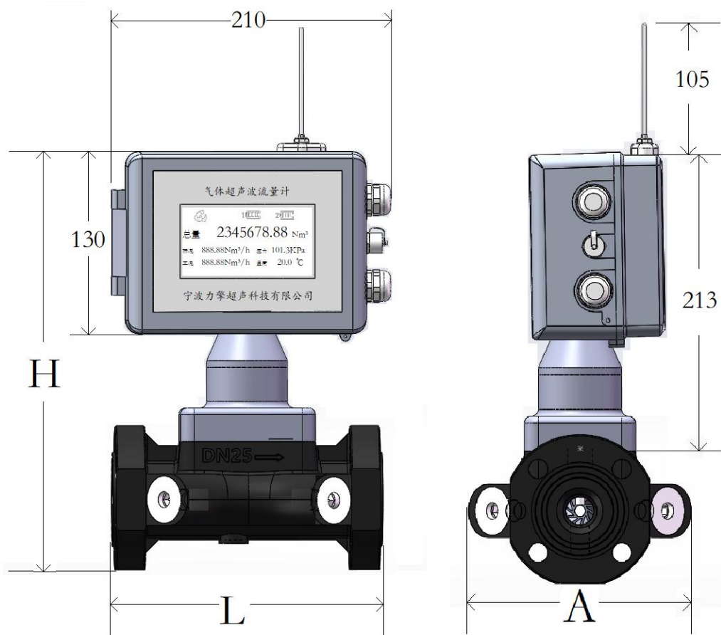
图4 LQUA 气体超声流量计（双声道）外形尺寸图
