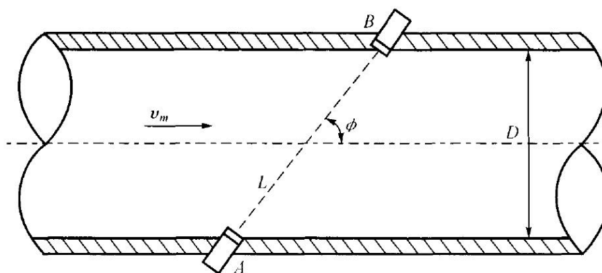
图 1 通用示意图
